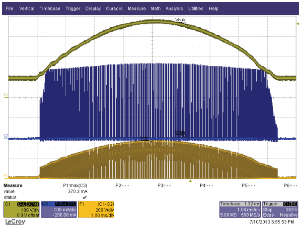
图15 – 265 VAC, 50 Hz, 额定 V_{LED} 负载 F1 (橙色): V_{D-S} , 200 V/格 Ch1 (黄色): V_{D-G} , 100 V/格 Ch3 (蓝色): I_{DRAIN} , 100 mA/格 时间量程: 1 ms/格
