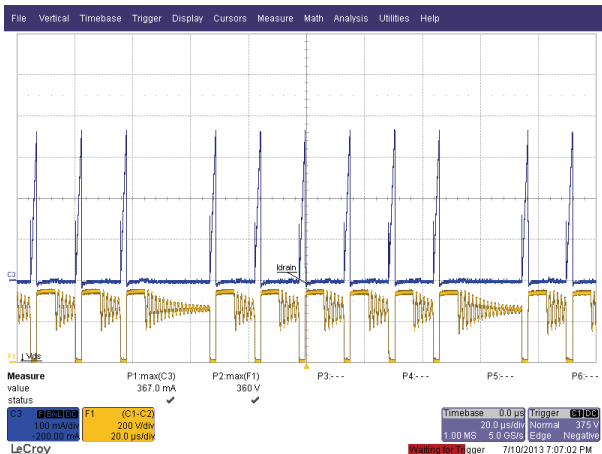
图17 – 265 VAC, 50 Hz, 额定 V_{LED} 负载 F1 (橙色): V_{D-S} , 200 V/格。 Ch3 (蓝色): I_{DRAIN} , 100 mA/格 时间量程: 20 \mu s/格
