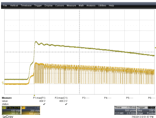
图41 – 差模振铃浪涌，2500 V/0°记录的 漏极峰值电压为404 V Ch1: V_{BULK} , 100 V/格 F1: V_{DRAIN} , 200 V/格 时间量程: 500 \mu s/格
