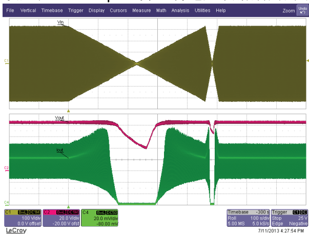
图36 – 电压跌落测试，1 V/秒和10 V/秒。 电源能够正常操作，而无人任何故障和闪烁。230 V - 0 - 230 V Ch1: V IN ，100 V/格 Ch1: V OUT ，20 V/格 Ch3: I OUT ，20 mA/格 时间量程：100 s/格
