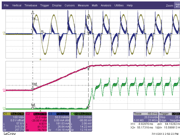
图23 – 230 VAC, 50 Hz, 额定 V_{LED} 负载
