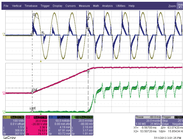
图25 – 265 VAC, 50 Hz, 额定 V_{LED} 负载
