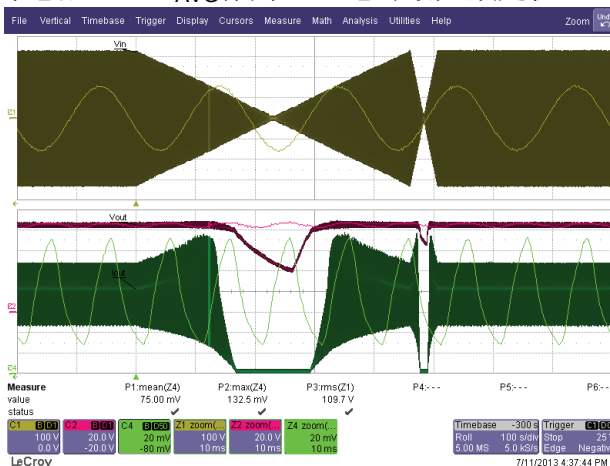
图37 – 电压跌落测试，1 V/秒和10 V/秒。 电源能够正常操作，而无人任何故障和闪烁。230 V - 0 - 230 V Ch1: V IN ，100 V/格 Ch1: V OUT ，20 V/格 Ch3: I OUT ，20 mA/格 时间量程：100 s/格
