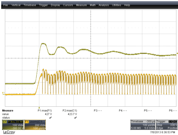
图39 – 差模输入浪涌，500 V/90°记录的 漏极峰值电压为427 V Ch1: V_{BULK} , 100 V/格 F1: V_{DRAIN} , 200 V/格 时间量程: 100 \mu s/格
