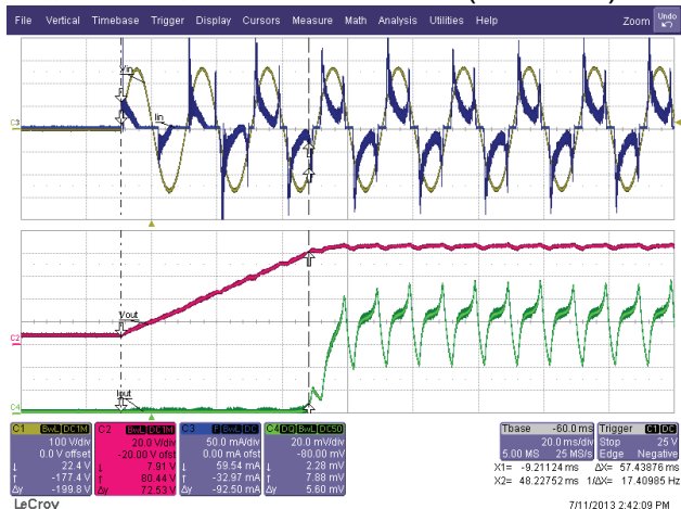
图22 – 190 VAC, 50 Hz, 额定 V_{LED} 负载
