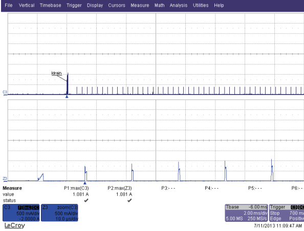
图18 – LYT0006D输出短路。265 VAC。 Ch3: I_{DRAIN} , 0.5 A/格 时间量程: 2 ms/格 Z4: V_{D-S} , 0.5 A/格 缩放时间量程: 10 \mu s/格
