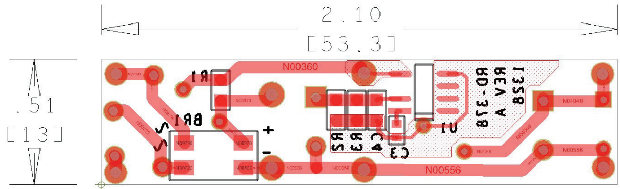
图6 - 印刷电路板布局 (底视图)
